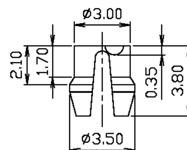
DETAIL Y
