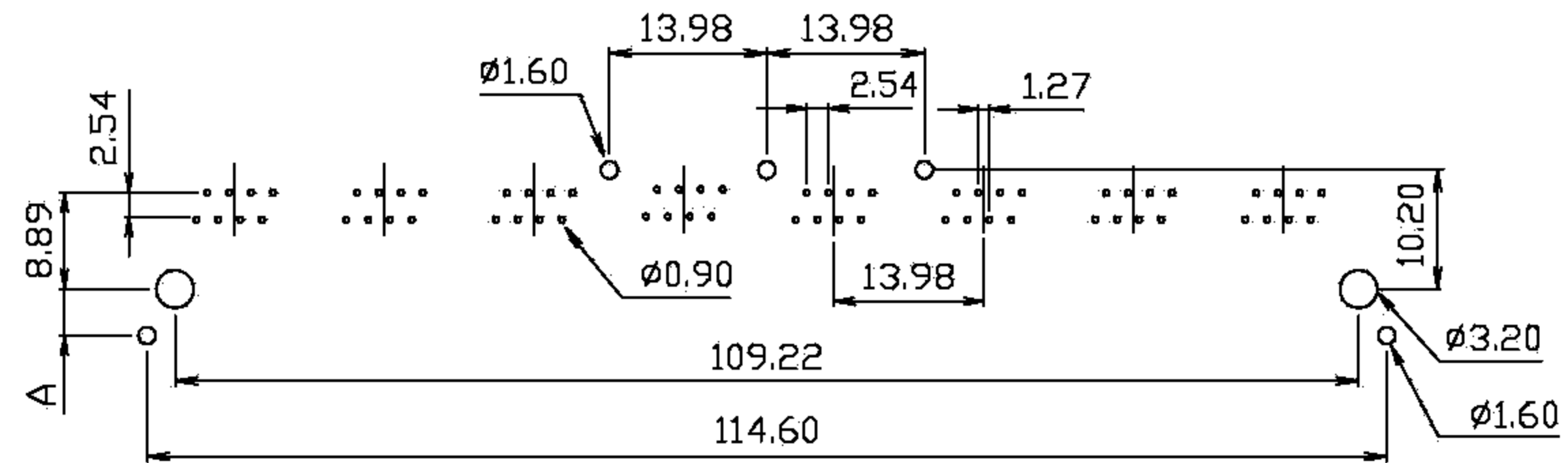
DETAIL Y
