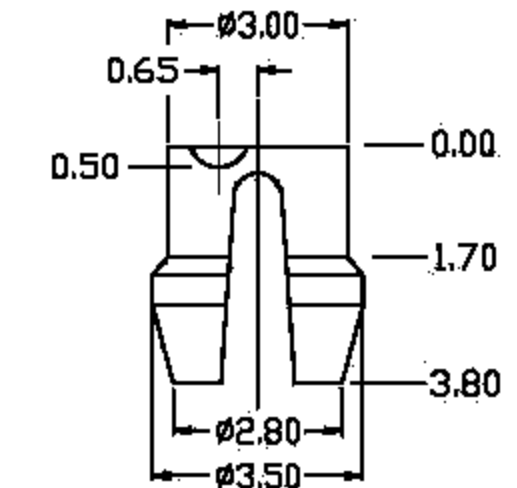
DETAIL Y
