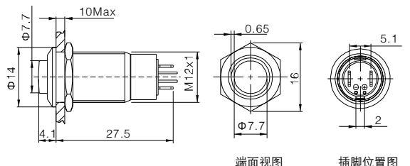
端面视图
