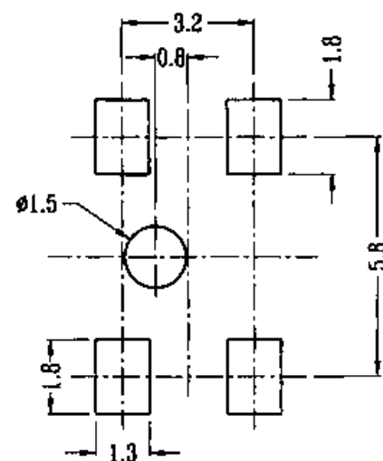
P.C.B. LAYOUT
