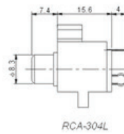
RCA-304L
