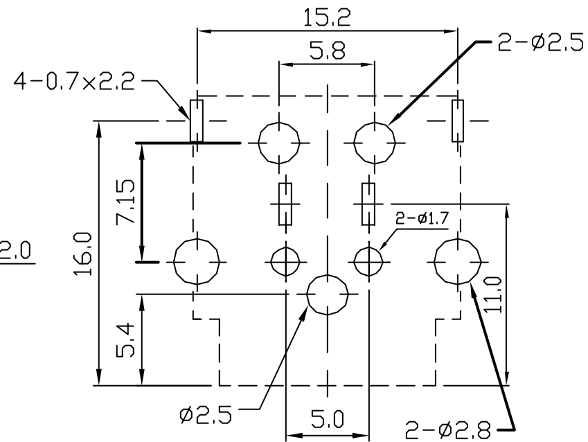
P.C.B LAYOUT(±0.1) (BOTTOM VIEW)
