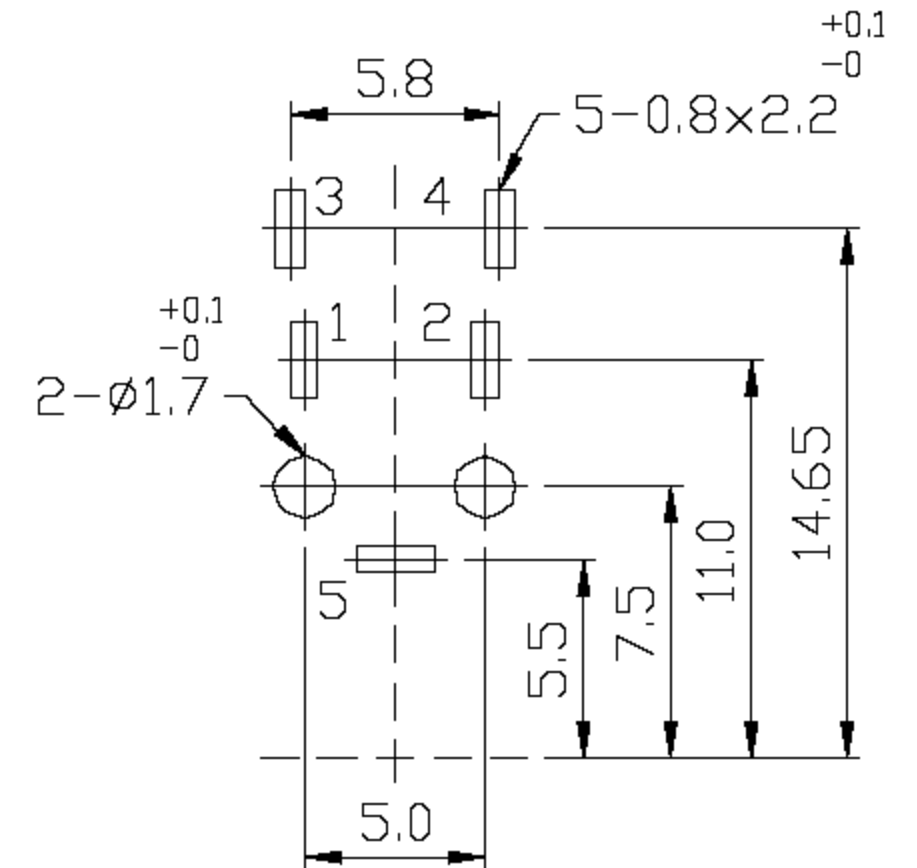
P.C.B LAYOUT(±0.1) (BOTTOM VIEW)
