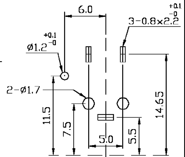
P.C.B LAYOUT(±0.1) (BOTTOM VIEW)
