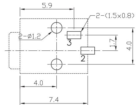
线路板开孔尺寸 P.C.B LAYOUT
